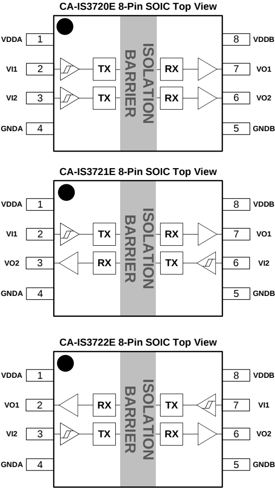
图 6-1 CA-IS372xE SOIC8 脚窄体封装顶部视图
